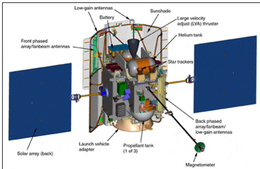
Устройство MESSENGER. Изображение с сайта messenger.jhuapl.edu
